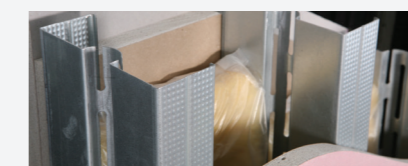
오메가 스테드 시스템 리질리언트 바와 결합하여 2시간 내화 및 1등급의 차음성능을 확보하며, 세대간 벽체 뿐만 아니라 세대 내에도 시공이 가능한 시스템
