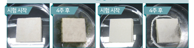
파이버락 0등급, 4주 후 곰팡이 성장 없음 CRC 2등급, 표면 곰팡이 10~30% 성장
